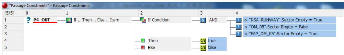
Slika 5.12. Prikaz grananja: a) uz izvođenje naredaba ako je uvjet zadovoljen, b) uz naredbe za oba slučaja ispunjenosti uvjeta, u programskom alatu CAST
