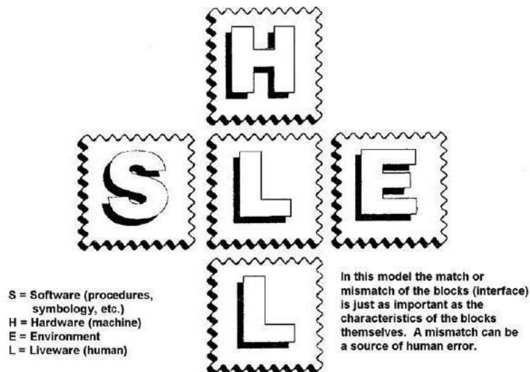
Slika 4 SHELL model
