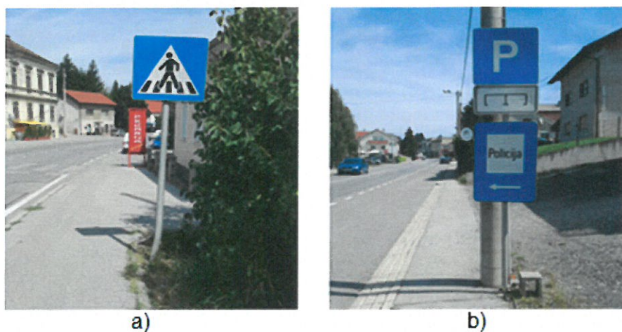
Slika 13. Primjer postavljanja znakova obavijesti na D3 u gradu Sveti Ivan Zelina: a) znak C02, b) znak C34 i C35
