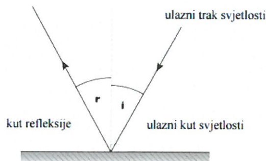
Slika 2. Zrcalna refleksija, [8]
