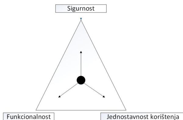
Slika 3. Trijada Sigurnost/Funkcionalnost/Jednostavnost.
