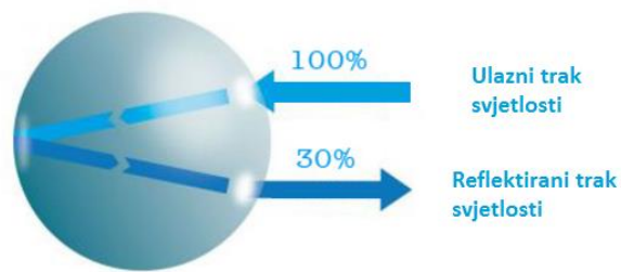
Slika 6. Sferična retrorefleksija
