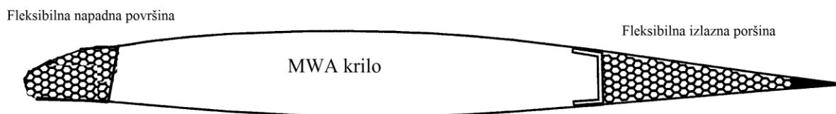
Slika 32. Primjer MWA krila
