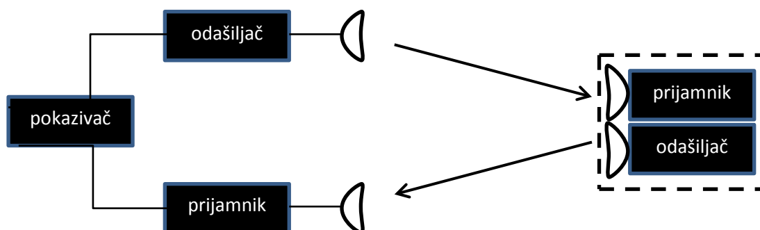
Slika 6. Blok shema radara sa aktivnim odjekom, [1]
