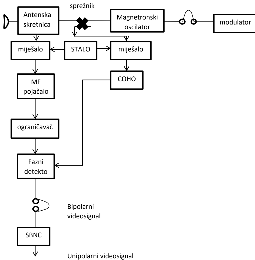
Slika 20. Blok shema Dopplerovog radara sa magnetronskim oscilatorom, [1]
