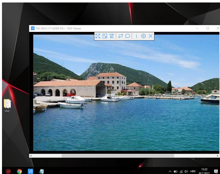
Slika 15: VNC sesija
