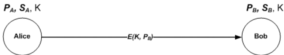
Slika 3: Asimetrična kriptografija
