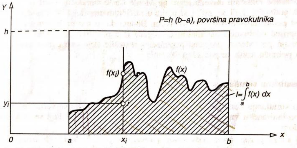
Slika 10. Računanje određenog integrala Monte Carlo simulacijom
