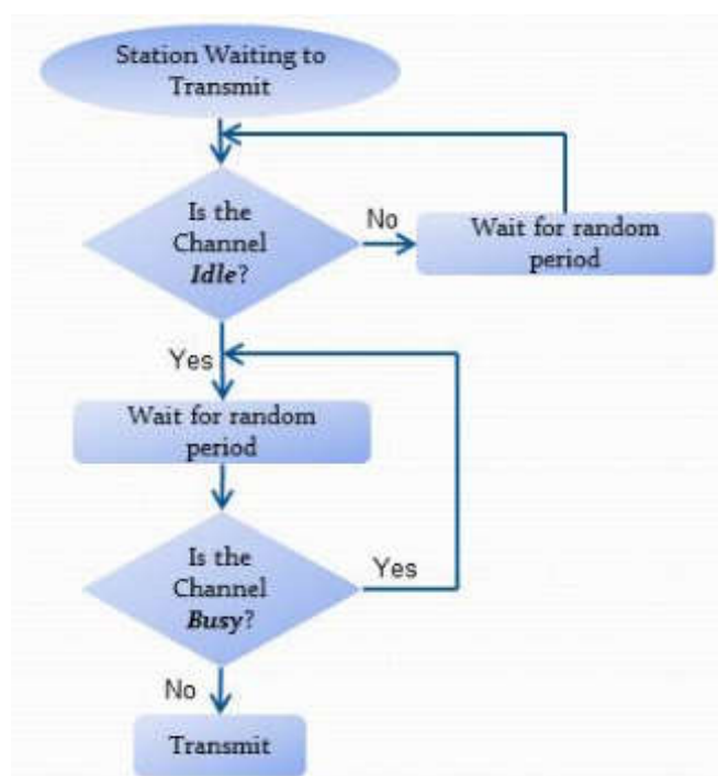
Slika 5. CSMA/CA mehanizam
