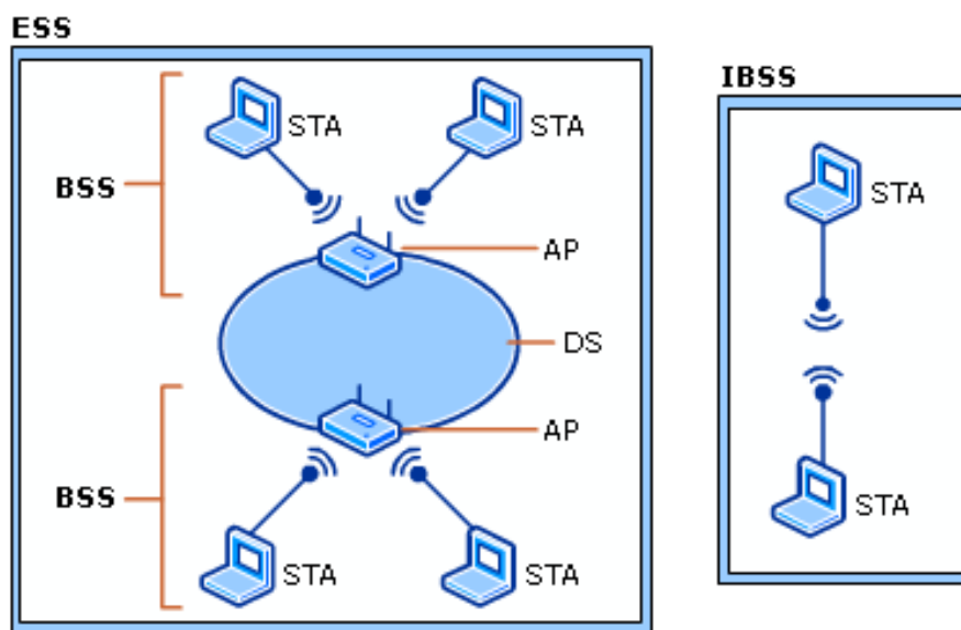
Slika 8. Arhitektura 802.11 mreže
