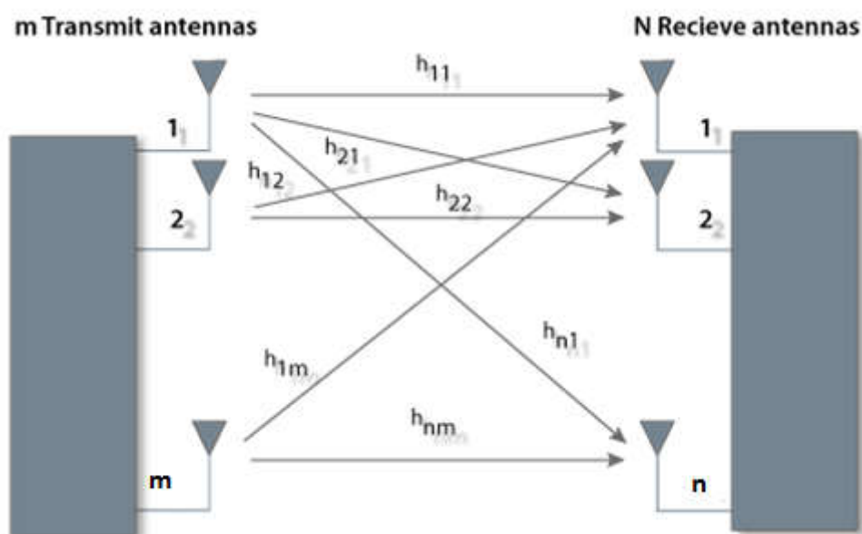
Slika 13. MIMO sustav
