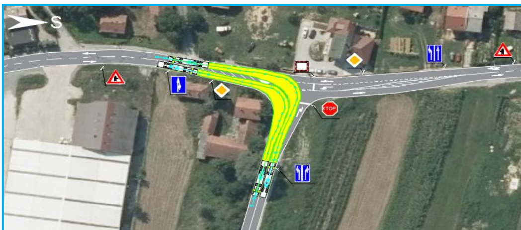
Slika 30. Trajektorija provoženja mjerodavnog vozila na raskrižju 2
