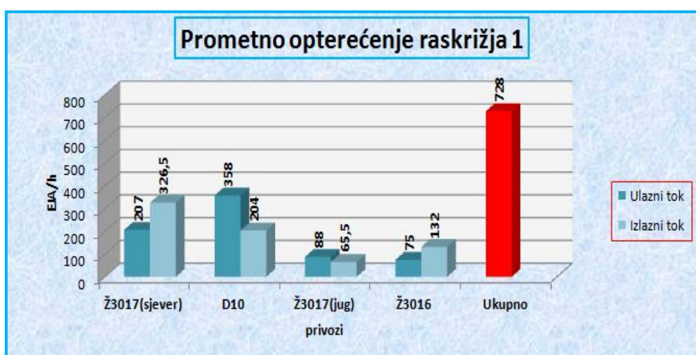
Grafikon 6. Prometno opterećenje pojedinih privoza i raskrižja 1 u popodnevnom vršnom satu
