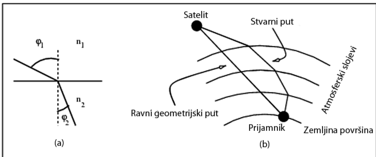
Slika 2: Utjecaj zemljine atmosfere na signal, [4]
