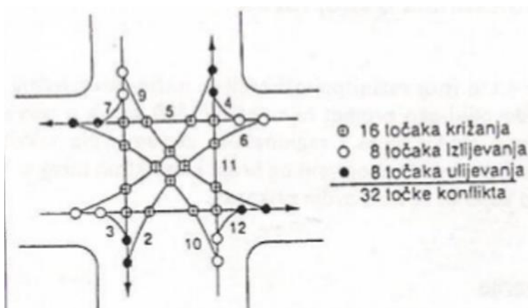
Slika 8. Konfliktni točke četverokrakog raskrižja
