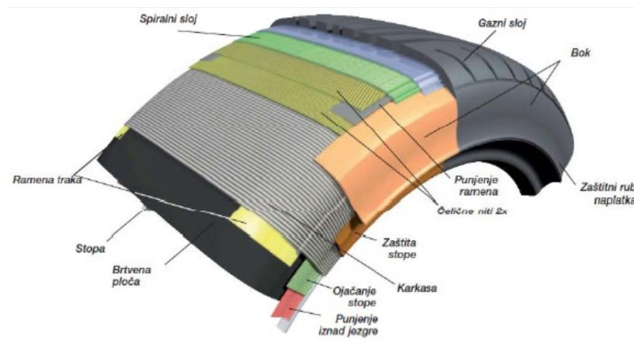
Slika 4. Presjek pneumatika
