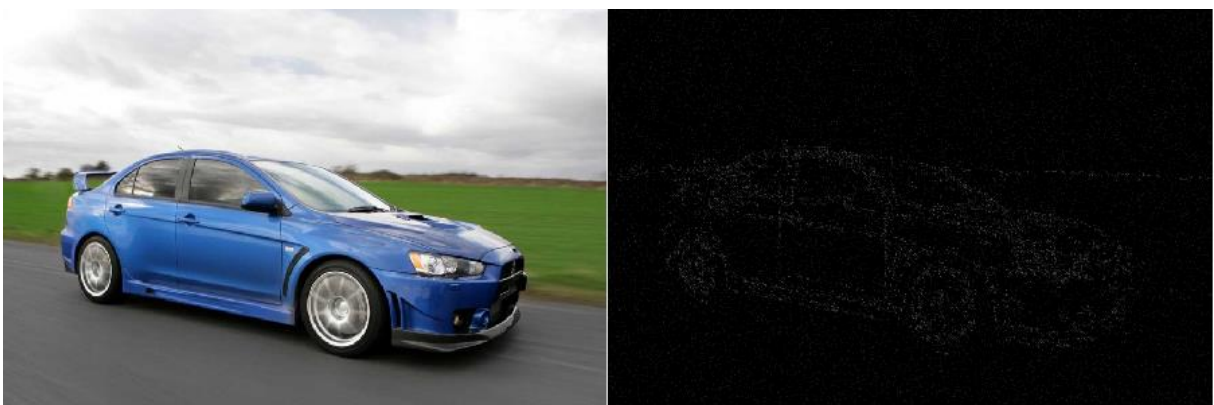
Slika 10. Kodiranje DynamicBattleSteg algoritmom, [13], [15]
