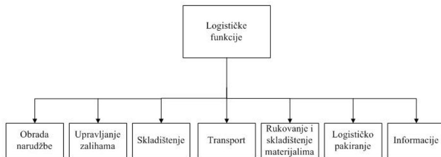
Slika 2. Logističke funkcije, [3]
