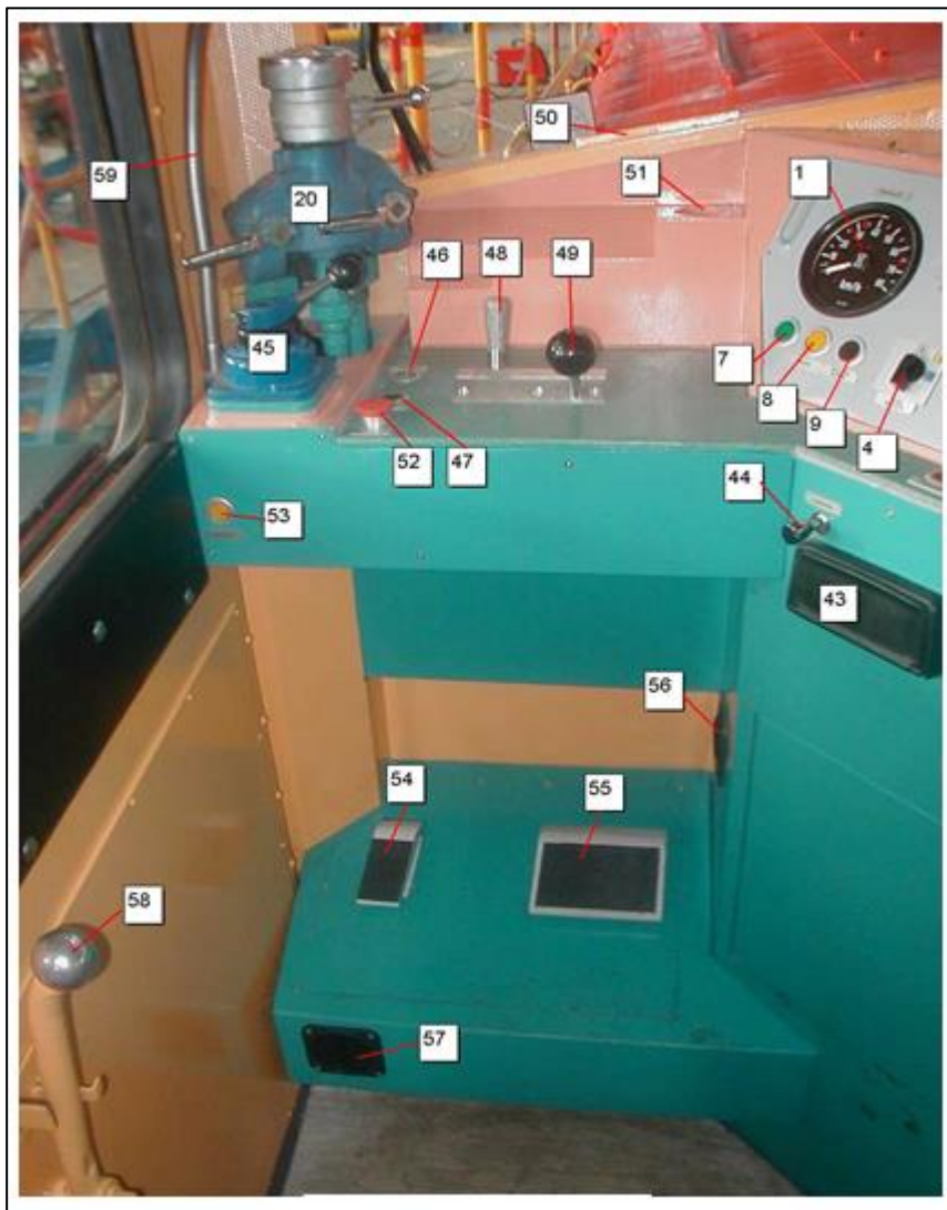
Slika 32. Upravljačnica 2
