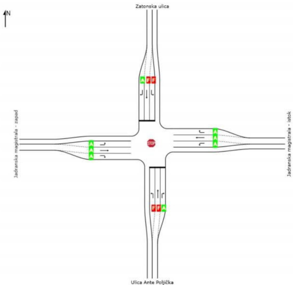
Slika 28. Prikaz razine usluge u raskrižju s trakovima za ubrzanje i usporenje
