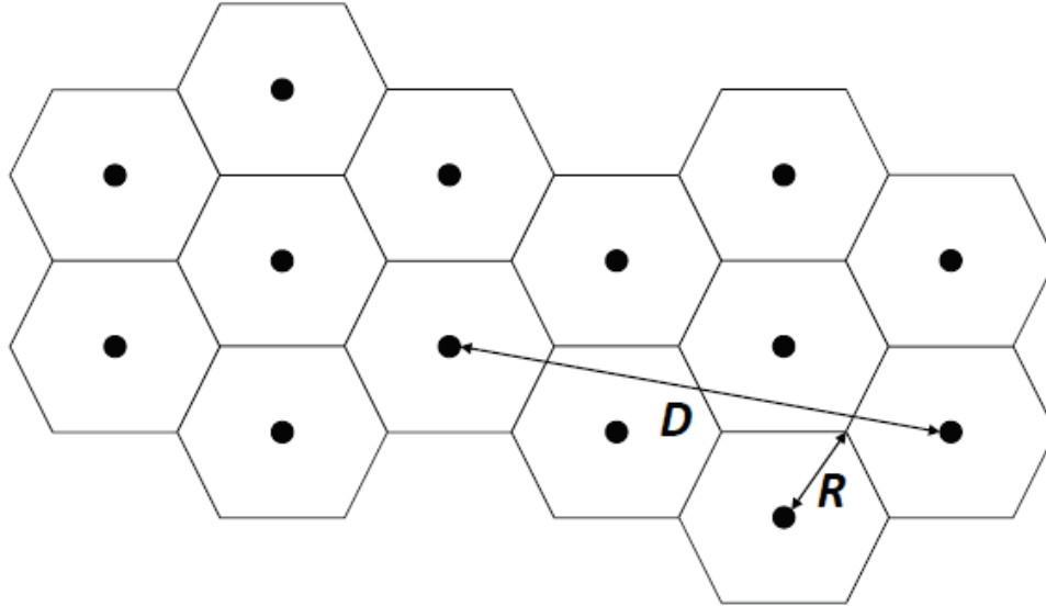
Slika 15. Čelijski koncept [22]
