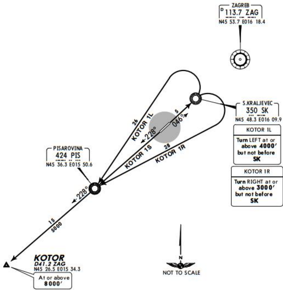
Slika 1. Procedure instrumentalnog odlaza sa zagrebačke zračne luke preko odlazne točke KOTOR [4]
