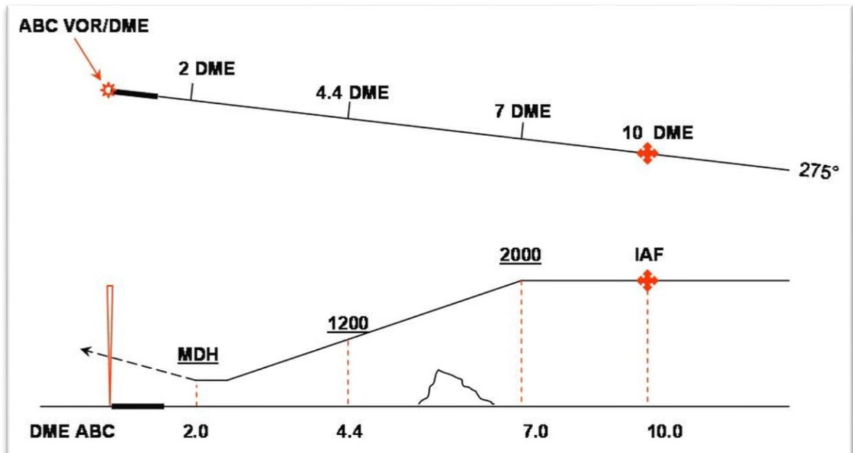
Slika 3. Shematski prikaz nepreciznog slijetanja
