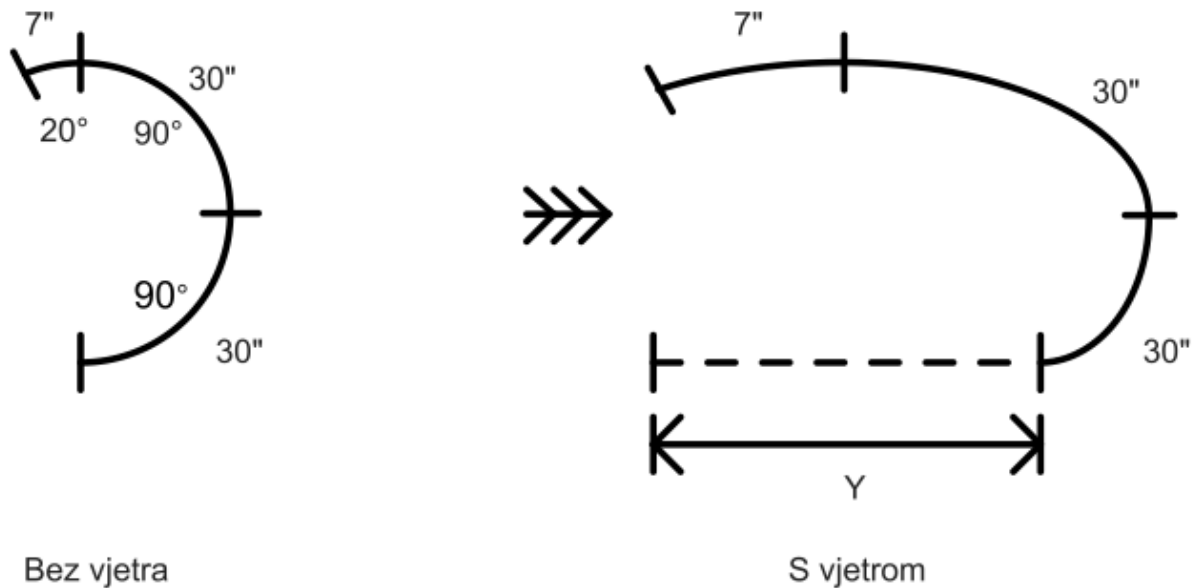
Slika 21. Utjecaj vjetra na zaokret od 200°
