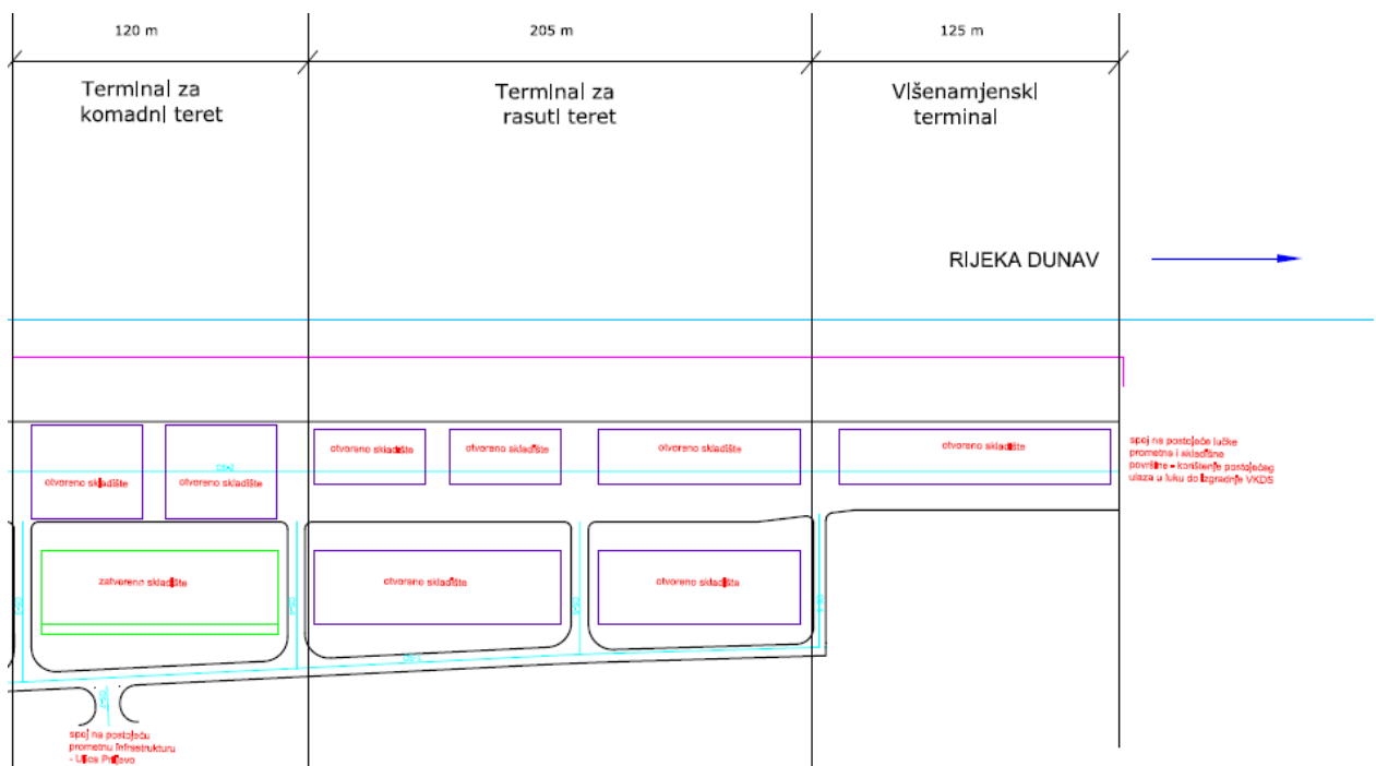
Slika 14. Luka Vukovar shema prometnih i skladišnih površina
