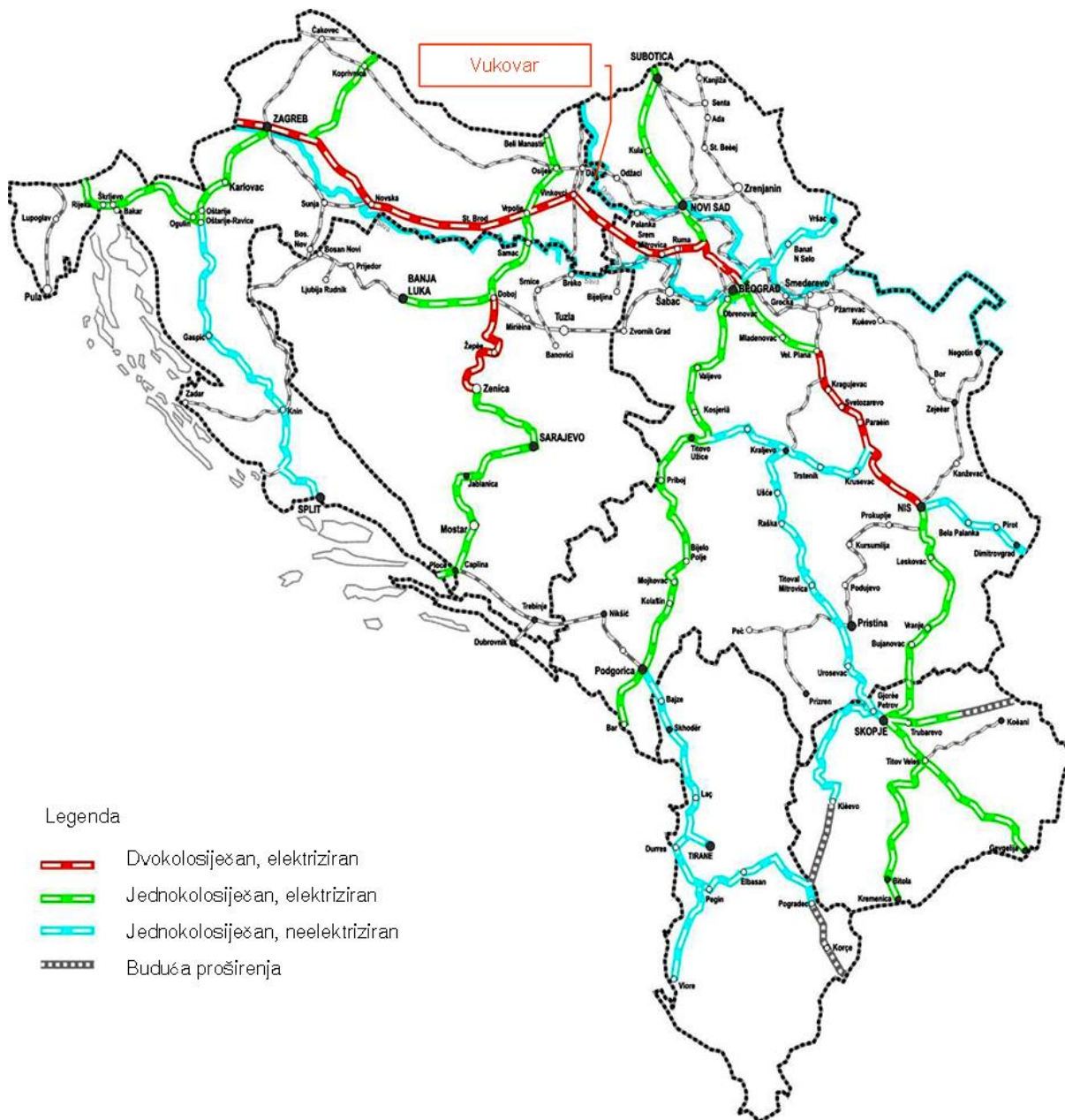
Slika 10. Aktualno tehničko stanje željezničke mreže
