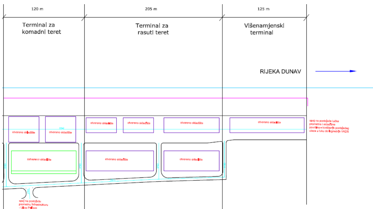
Slika 14. Luka Vukovar shema prometnih i skladišnih površina
