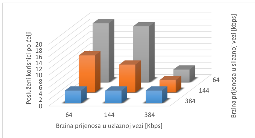
Grafikon 13. Broj posluženi korisnika po ćelji za asimetrični prijenos i opterećenje uzlazne veze od 80%,
