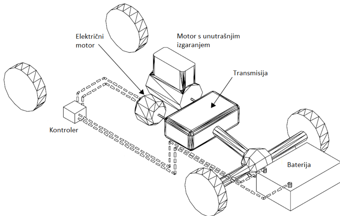
Slika 8. Shema paralelnog hibrida [2]
