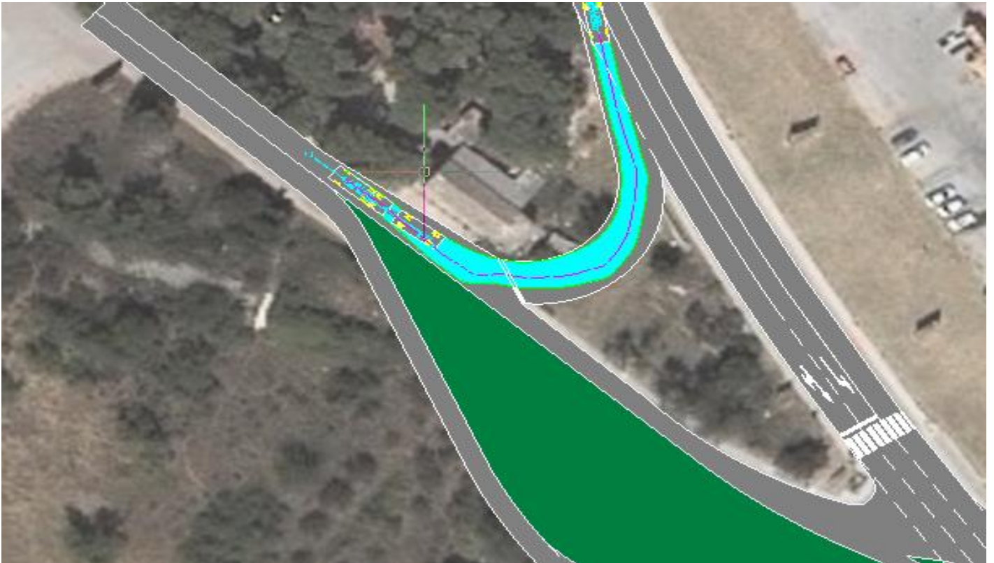
Slika 19. Traektorije teretnog vozila (kamion s prikolicom) izrađene programskim alatom AutoTURN za četverokrako raskrižje
