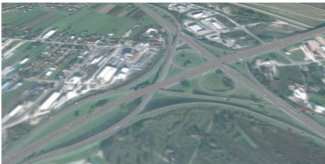
Slika 40. Prikaz stanja prometa na čvoru Lučko nakon implementacije odabranog varijantnog rješenja u programskom alatu PTV Vissim
