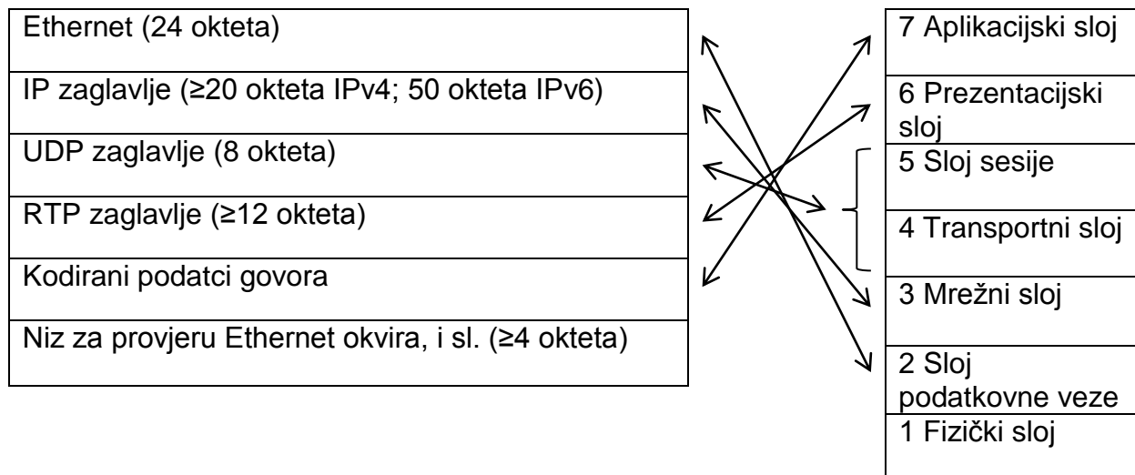
Slika 2. Dodavanje zaglavlja VoIP paketa. Preuzeto od [1].
