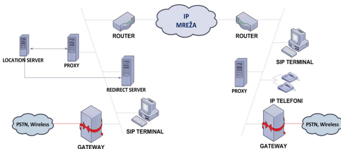
Slika 10. SIP arhitektura. Preuzeto od [11].
