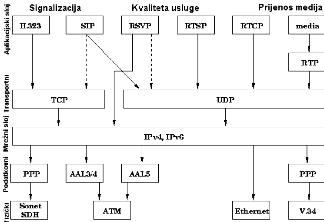
Slika 8. VoIP protokoli kroz OSI referentni model. Preuzeto od [10].
