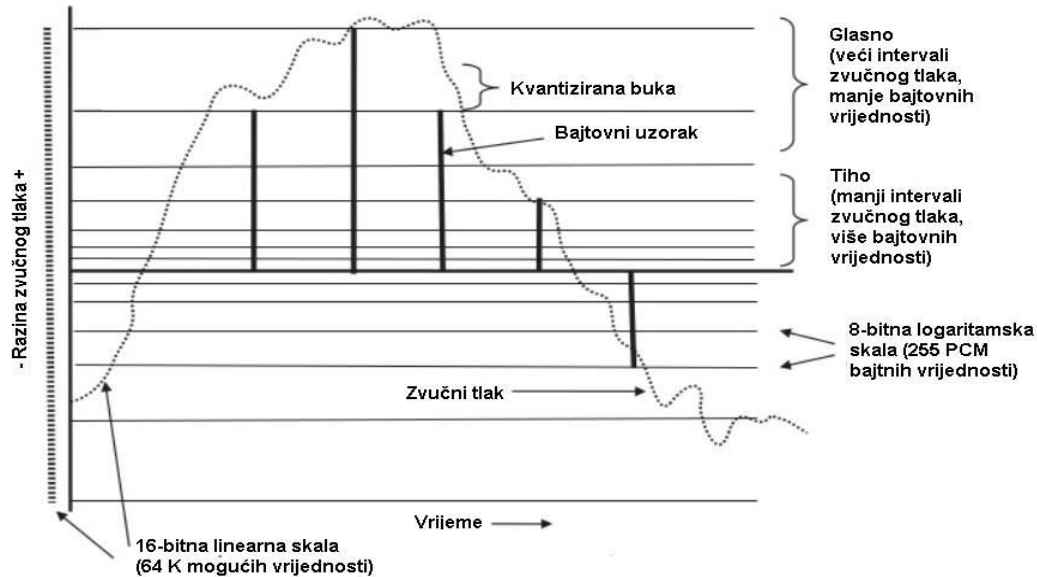
Slika 3. Kodiranje glasa. Preuzeto od [1].
