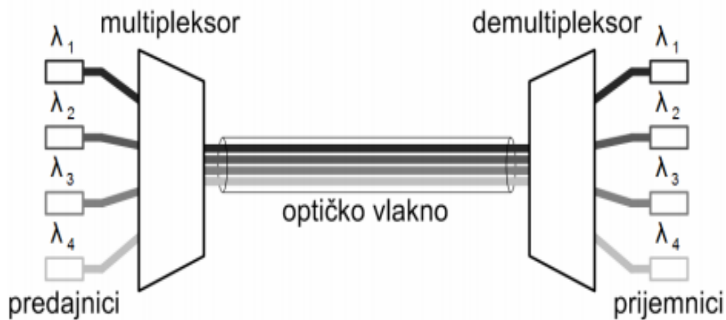
Slika 1. WDM sustav (multipleksiranje valnom podjelom)
