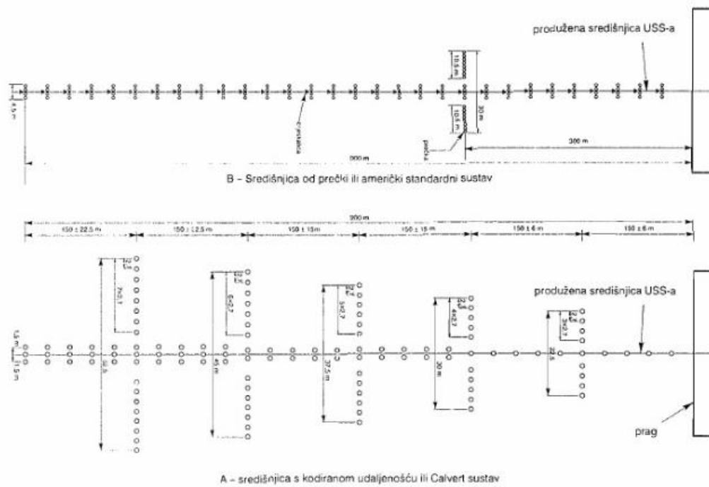
Slika 2. Američki standardni i Calvert sustav preciznog prilaza kategorije I, [3]
