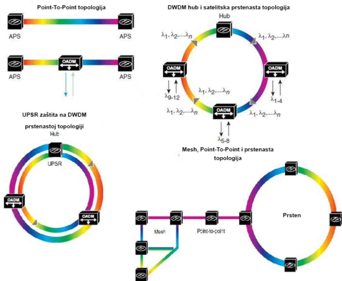
Slika 6.4, Metro topologije, [24]
