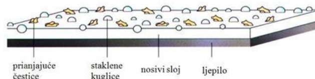
Slika 18. Neprofilirane oznake na kolniku izrađene trakom
