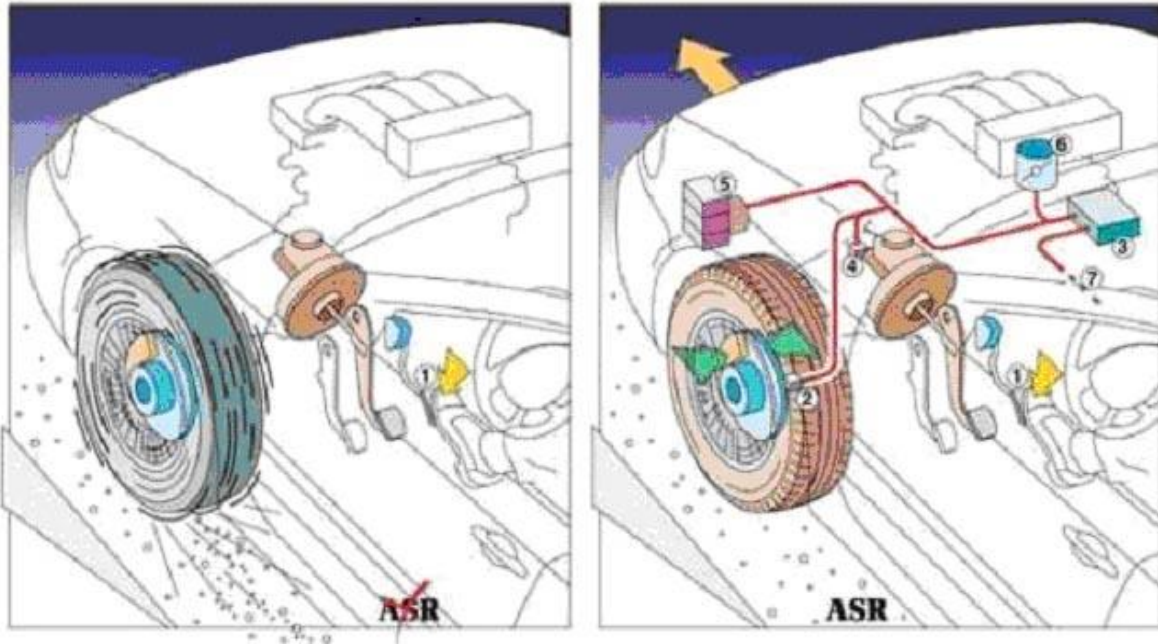
Slika 11. Sprječavanje proklizavanja [22]
