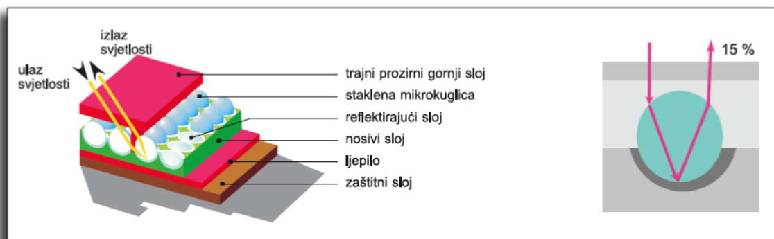
Slika 4. Materijal Klase II – High Intensity Grade Izvor:[6]
