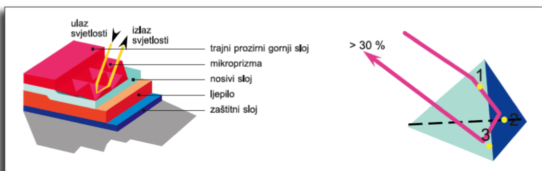
Slika 5. Materijal Klase III – Diamond Grade Izvor:[6]
