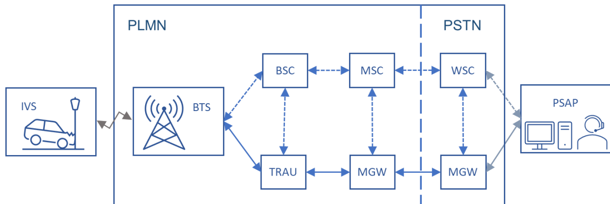
Slika 5. Komponente telekomunikacijskih mreža i njihova međusobna povezanost. Izvor: [7]
