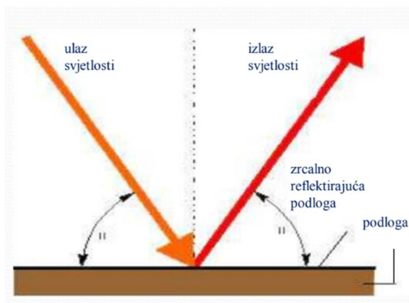
Slika 7. Zrcalna refleksija
