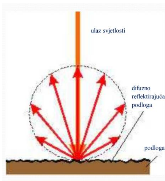
Slika 8. Difuzna refleksija
