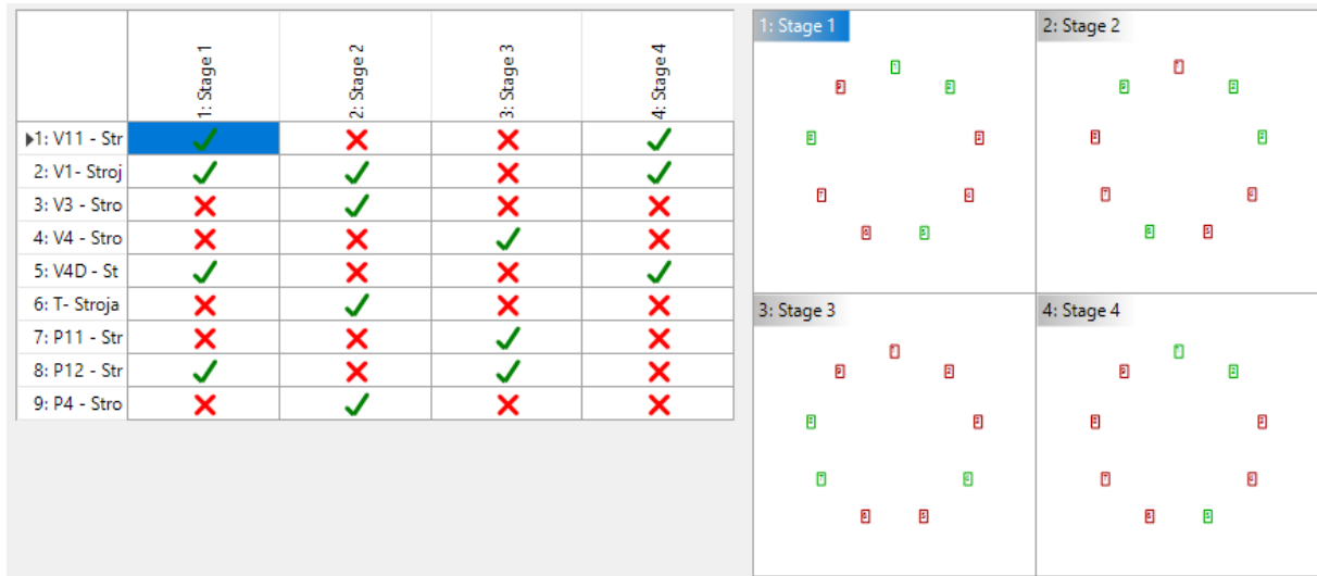
Slika 36. Prikaz rasporeda faza i pripadajućih signalnih grupa na raskrižju Strojarska ulica – Vukovarska ulica
