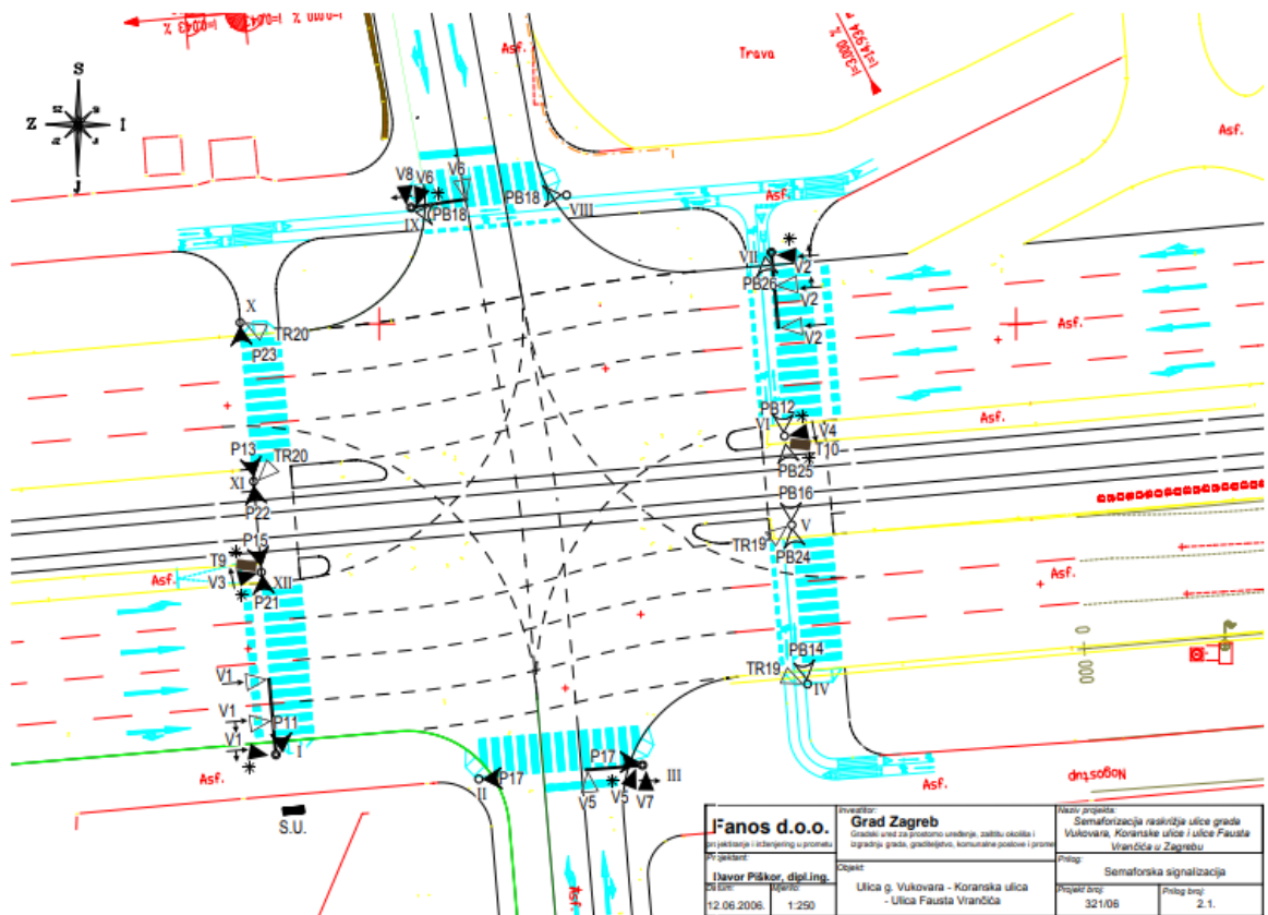
Slika 17. Prikaz vanjske situacije semaforizacije na raskrižju Koranska ulica – Vukovarska ulica
