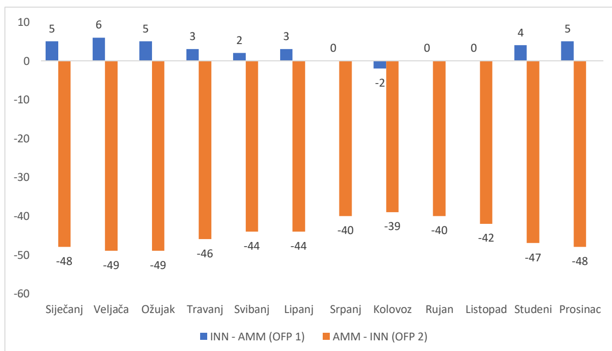
Slika 30. Graf 2 - Promjene vrijednosti vjetro kroz godinu na relaciji INN – AMM – INN
