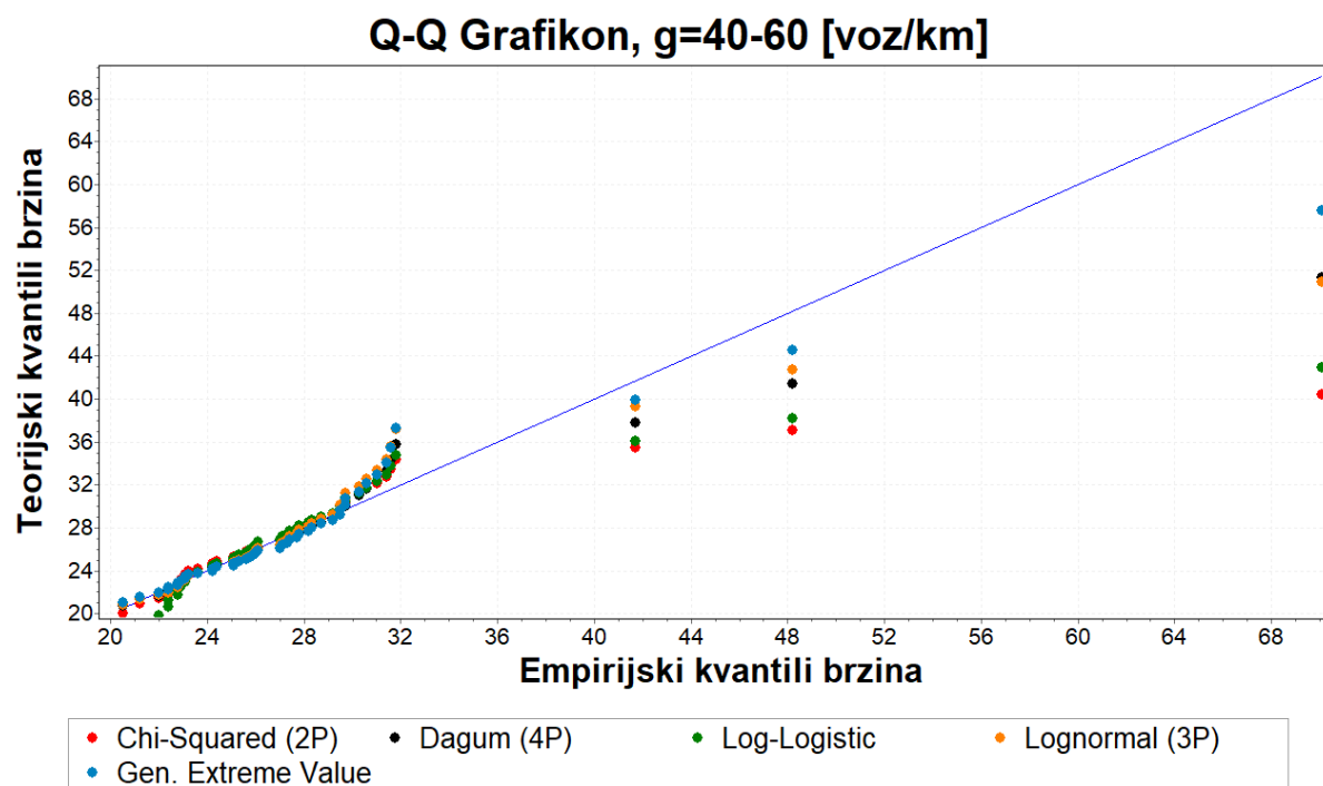
Grafikon 75. Prikaz odnosa vrijednosti kvantila brzina empirijskih i odabranih teorijskih razdioba ocijenjenih prikladnima za opis varijabilnosti parametra brzine prometnog toka u intervalu vrijednosti gustoće prometnog toka od 40 do 60 voz/km/traku. Izvor: obrada autora u programskom okruženju EasyFit 5.6 Professional .
