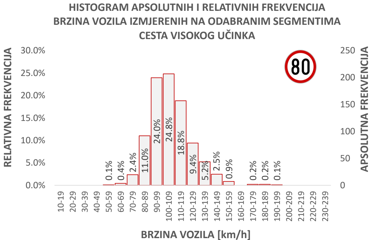
Grafikon 11. Empirijske razdiobe apsolutnih i relativnih učestalosti (frekvencija) izmjerenih vrijednosti brzina individualnih vozila u prometnom toku na odabranim segmentima cesta visokog učinka s ograničenjem brzine od 80 km/h, po definiranim statističkim razredima. Izvor: obrada autora.
