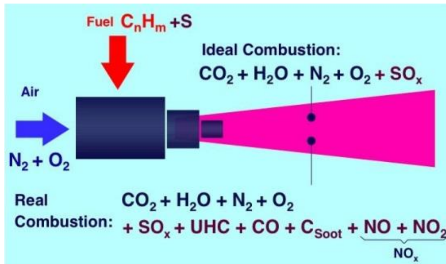
Slika 2 Produkti pri idealnom i stvarnom izgaranju [6]
