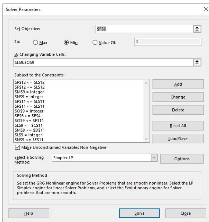
Slika 16. Prikaz excel solver prozora za definiranje ograničenja
