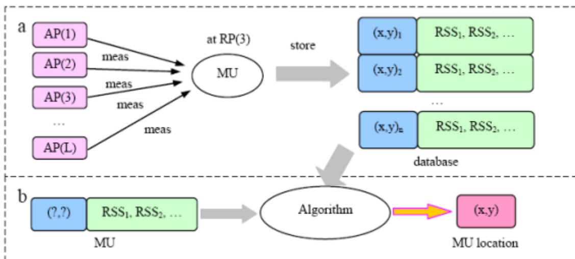
Slika 20. Metoda figerprinting, [18]
