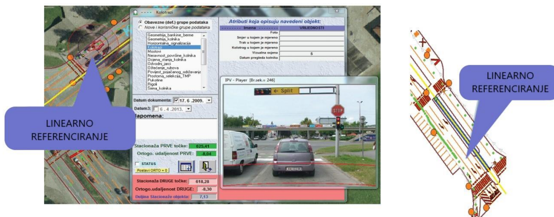
Slika 19. Linearno referenciranje podržano georeferenciranim videozapisom.
