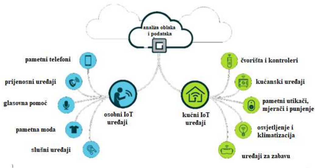
Slika 12. Mogućnosti IoT
