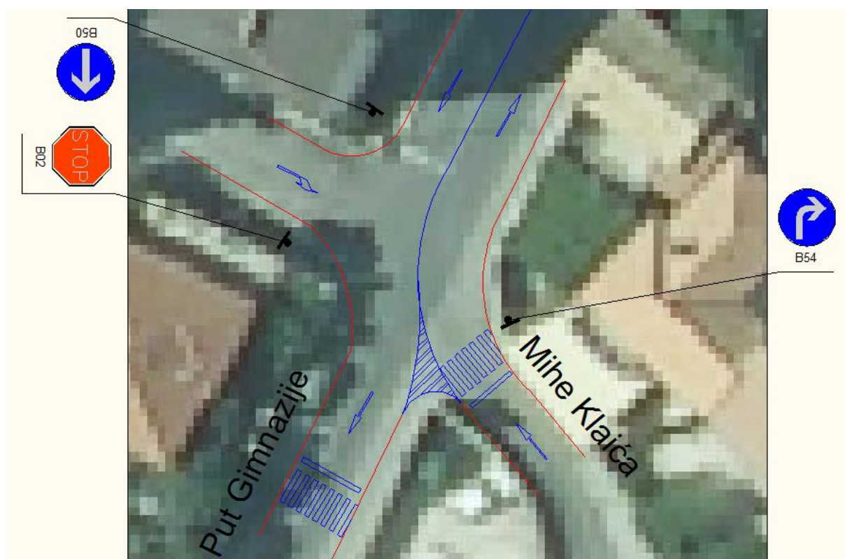
Slika 14. Idejno prometno rješenje raskrižja ulice Put gimnazije i ulice Mihe Klaića
