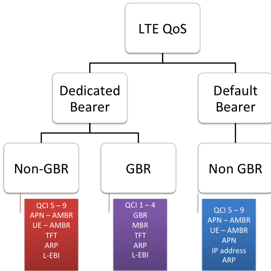
Slika 9. Podjela nositelja [9].
