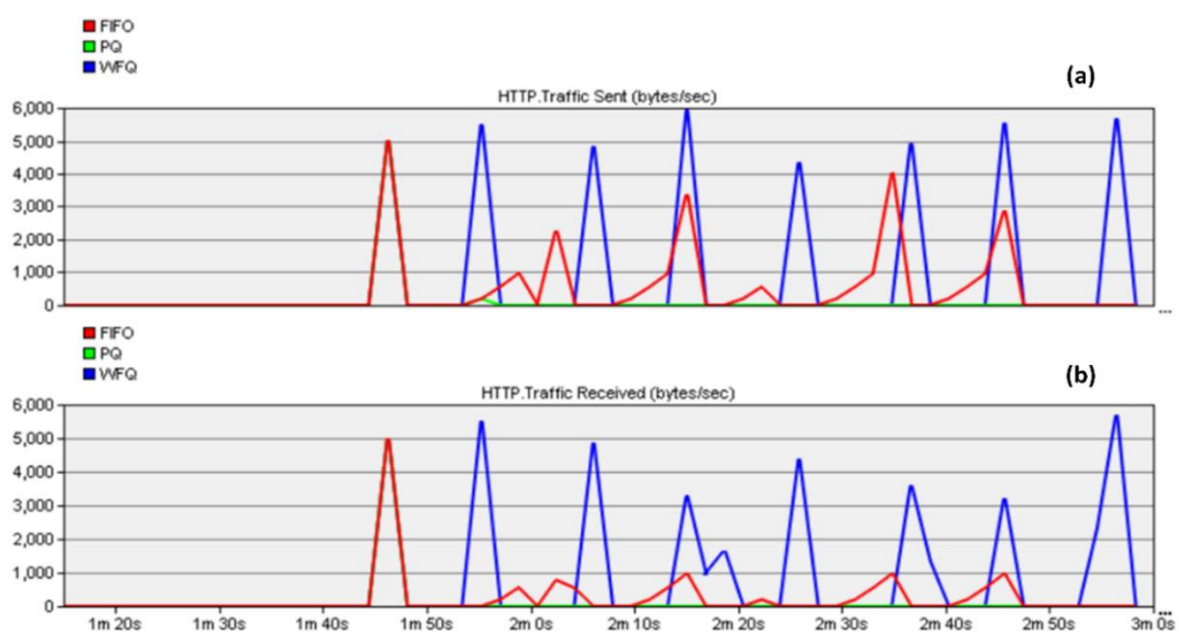
Graf 2. Veličina poslanog (a) i primljenog (b) prometnog toka HTTP aplikacije za FIFO, PQ i WFQ metode posluživanja
