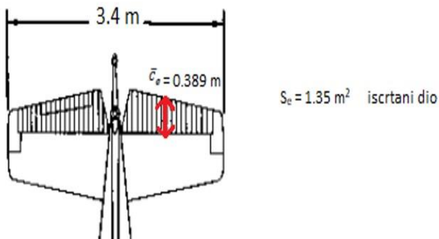
Slika 38. Geometrija repa
