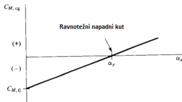
Slika 12. Krivulja koeficijenta momenta s pozitivnim nagibom [1]
