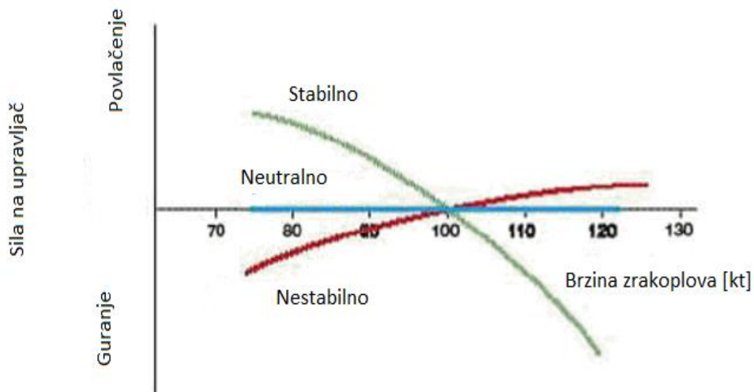
Slika 34. Primjer izgleda F/V grafičari za pozitivnu stabilnost, neutralnu stabilnost i nestabilnost [8]
