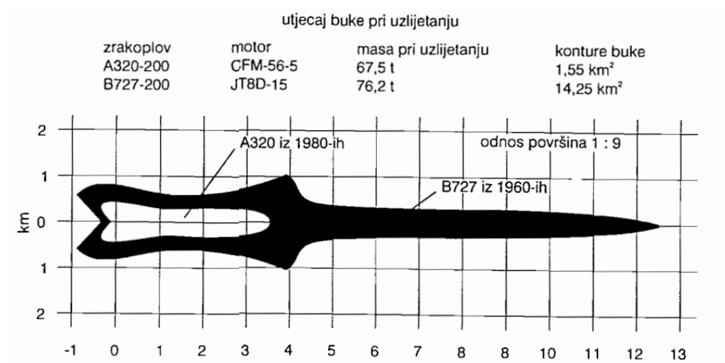
Slika 1. Različiti utjecaj zrakoplova na stvaranje buke
