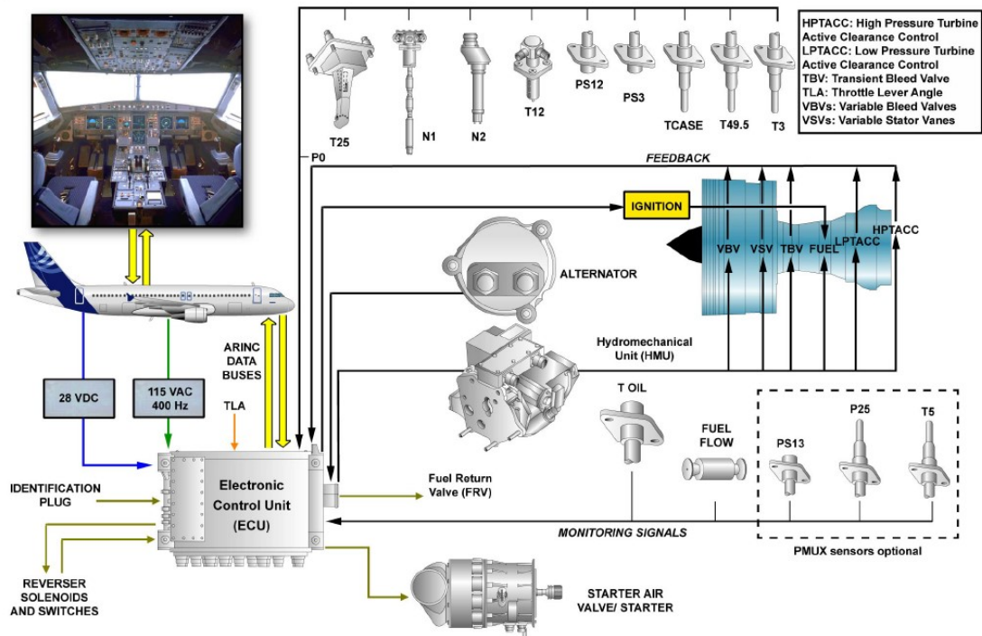
Slika 9. FADEC mreža [18]
