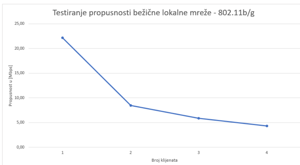
Slika 24: Linijski graf o ovisnosti propusnosti i broja trenutno spojenih klijenata – 802.11b/g
