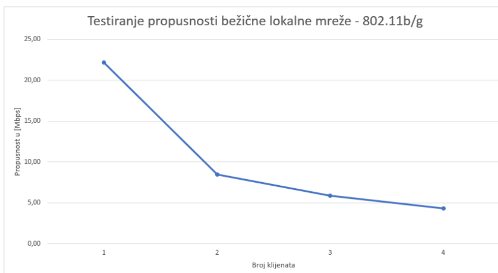
Slika 24: Linjski graf o ovisnosti propusnosti i broja trenutno spojenih klijenata – 802.11b/g
