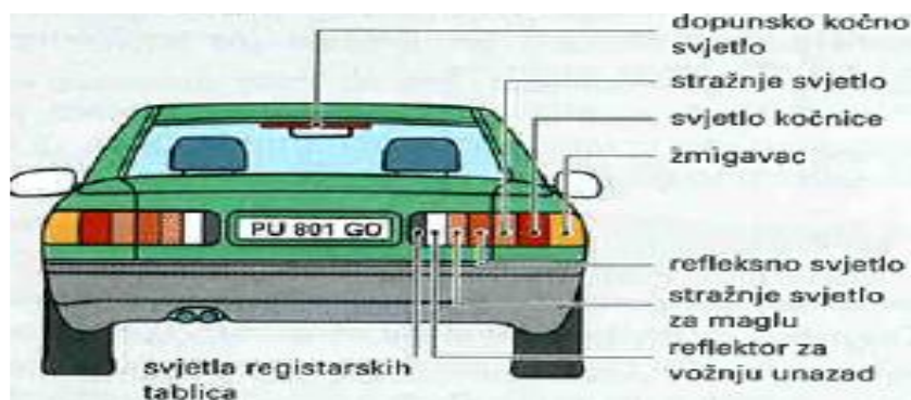
Slika 5.4. Svjetla na stražnjoj strani vozila
