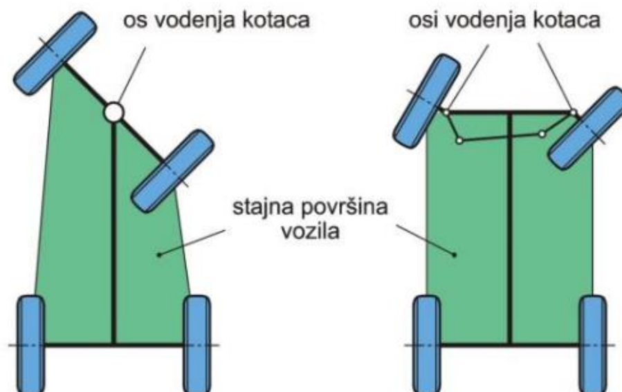
Slika 13. Upravljanje zakretnom oplonom i zakretanjem smjernih površina
